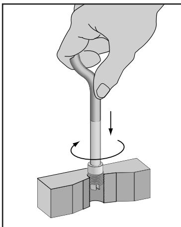
Inserire il filetto riportato Installing wire insert
